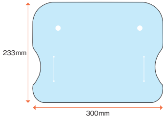
平面図 (表面)
